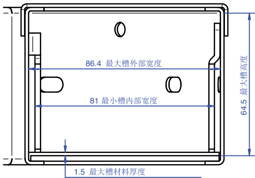
槽入口详情
