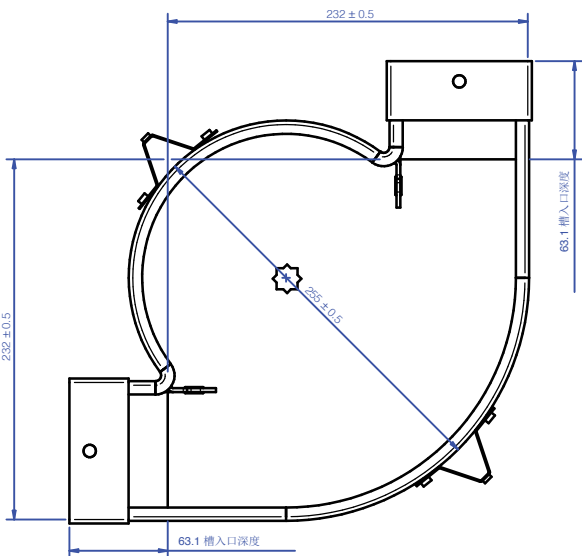
转角轮尺寸
