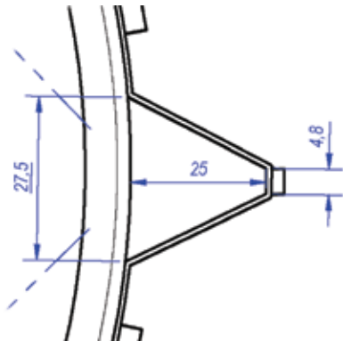
适配转角轮的最大腿架
